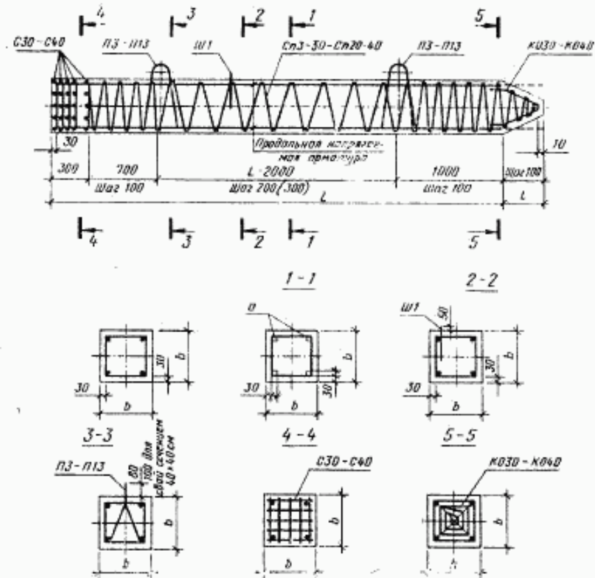
а—зона расположения продольной арматуры при 3 и более проволок, канатов.
